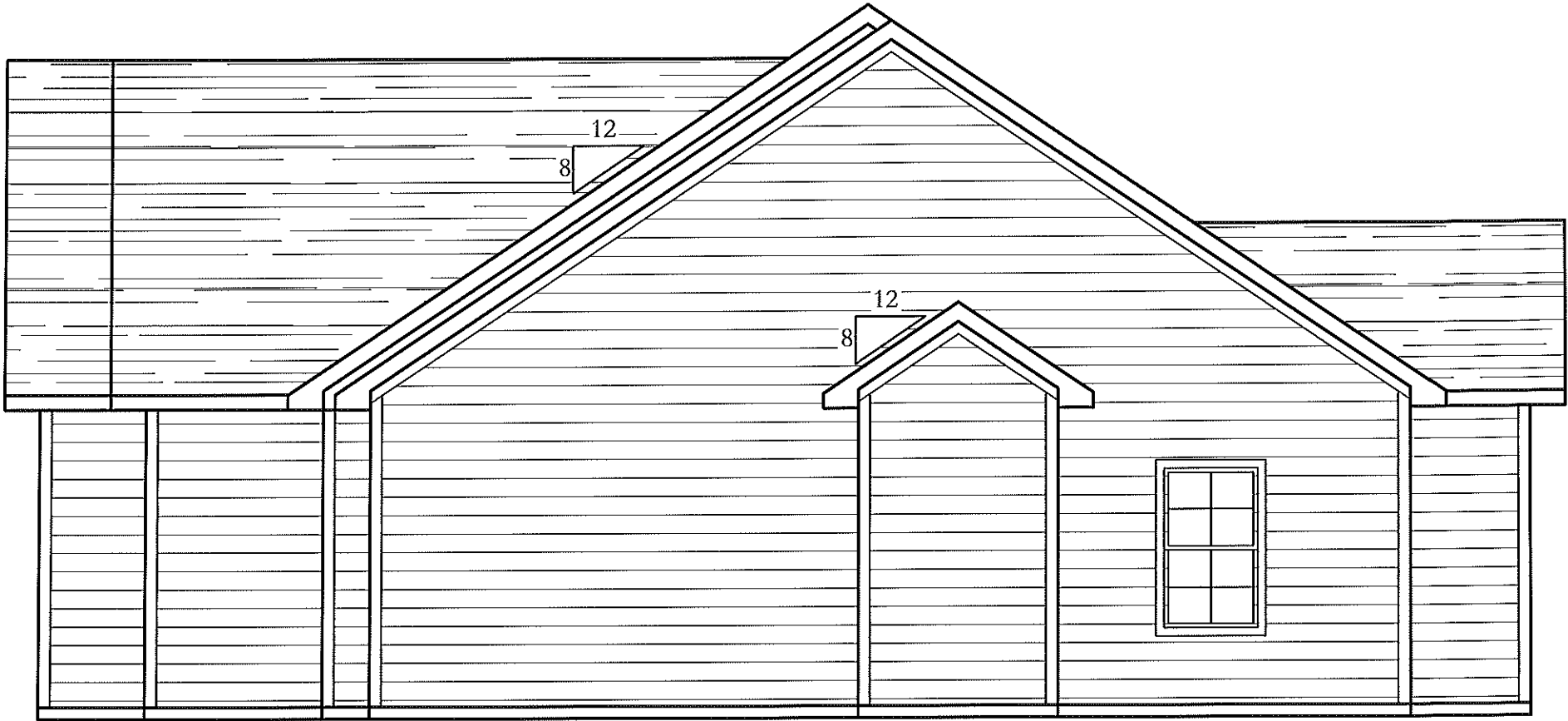
RIGHT ELEVATION
